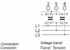
Esquemas de conexión Connections diagrams
