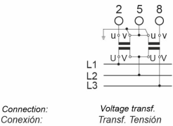
Esquemas de conexión Connections diagrams
