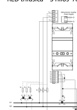
RED trifásica - 3 hilos- ARON
